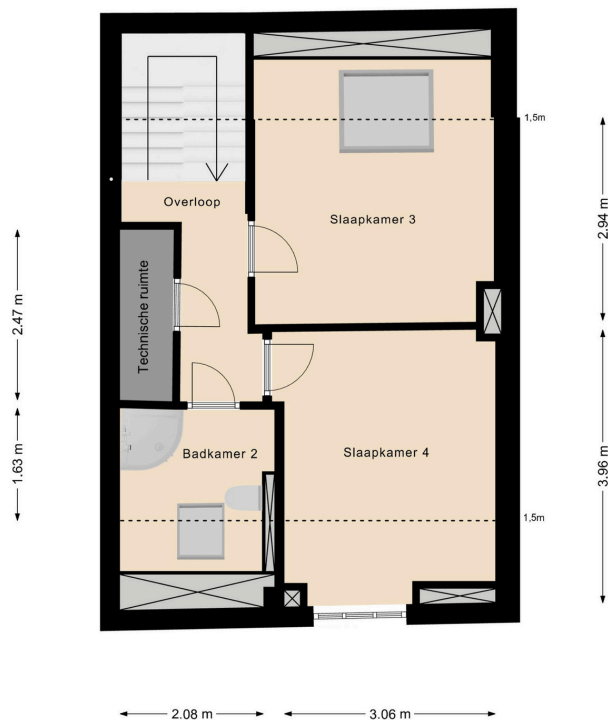
Tweede verdieping Stationsstraat 6, Schinnen
